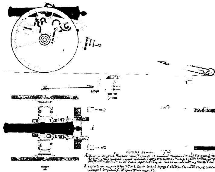
Полковая 3-хъ фунт. пушка. съ черт. хран. въ Истор. Артл. Музеѣ.
